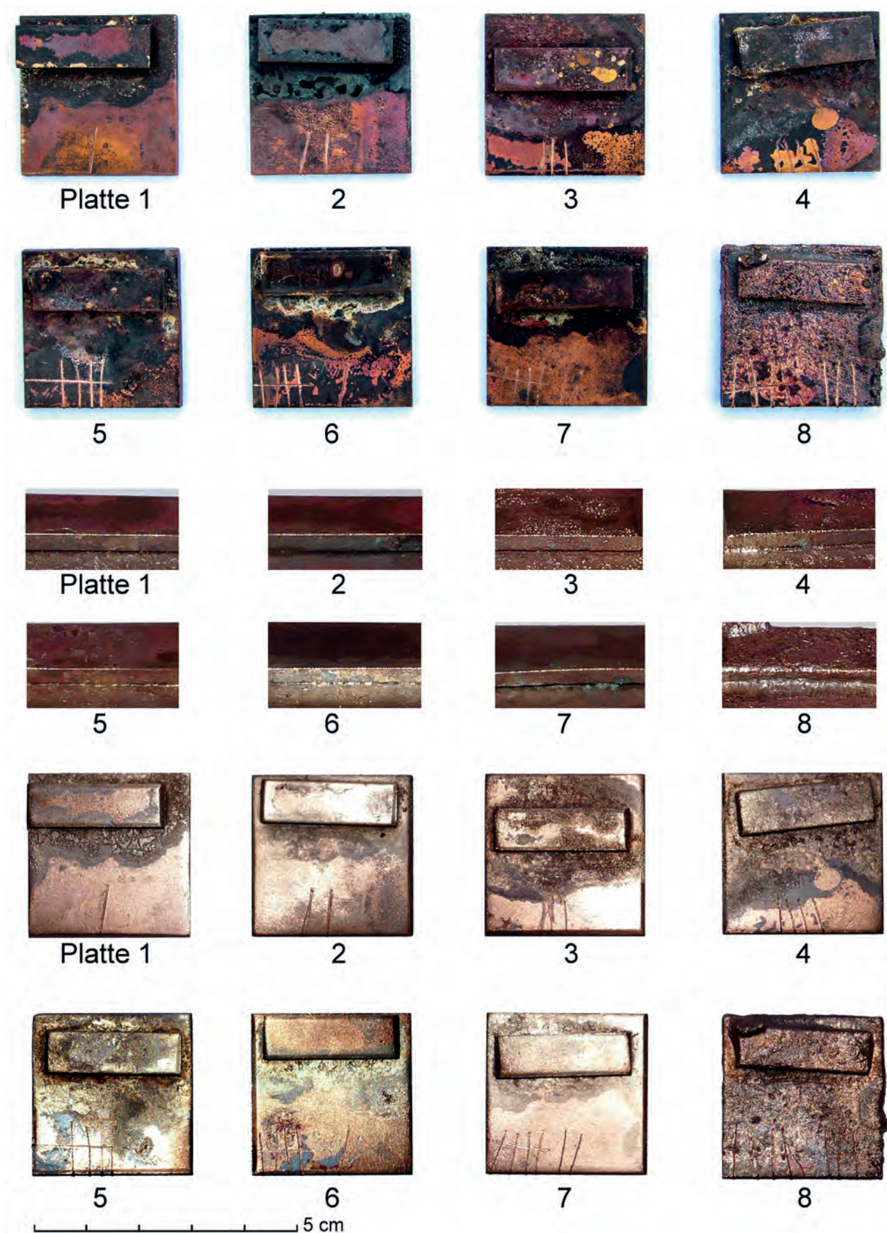
Abb. 10 Die Platten 1–8 einige Monate nach dem Lötversuch: obere Doppelreihe: mit Wasser gebürstet; untere Doppelreihe: mit Kratzwasser gebürstet; mittlere Doppelreihe: Details der Lötstellen in doppelter Grösse.
