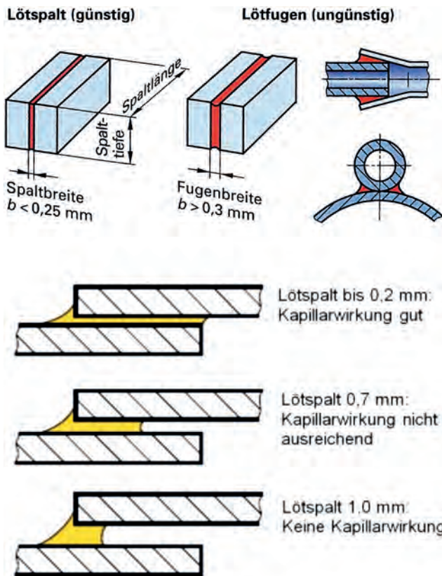
Abb. 1 Lötspalt und Lötfläche.
